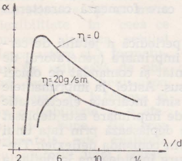
Fig. 4.55. Variația factorului de creștere \alpha în funcție de raportul \lambda/d și de vâscozitatea \eta a cernelii.
