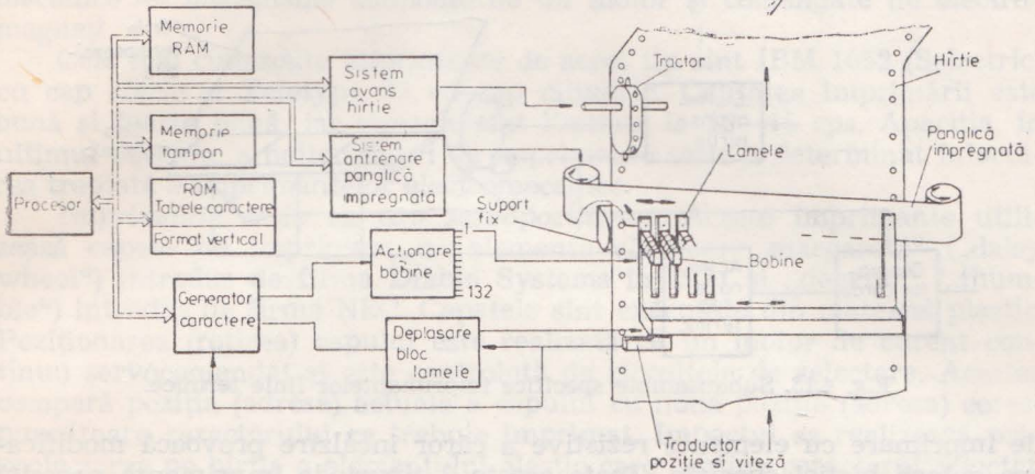
Fig. 4.11. Structura unei imprimante linii cu impact matricială.
