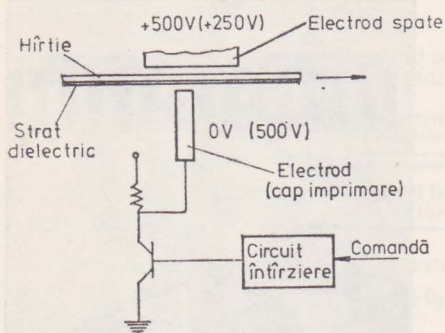
Fig. 4.44. Imprimarea electrostatică — schema stației de încărcare electrostatică a hârtiei.
