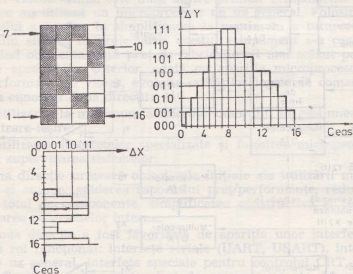
Fig. 7.10. Generarea caracterului R pe o matrice 4×7.
