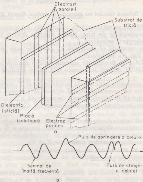
Fig. 7.5. Schema panoului cu plasmă (a) și semnalul de comandă pentru panoul cu plasmă (b).
