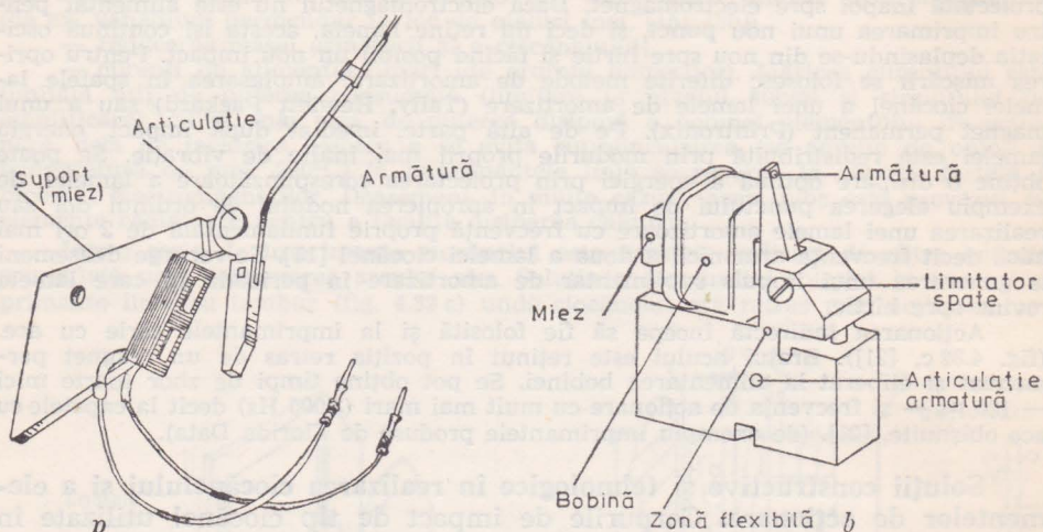
Fig. 4.34. Electromagneți de acționare a ciocănelului: a — imprimanta CDC 5403; b — imprimantele Documation.
