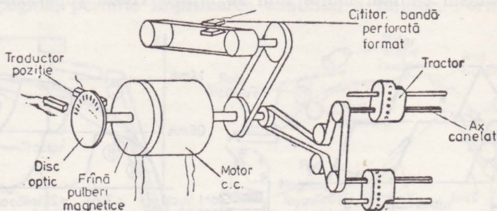
Fig. 4.81. Acționare cu motor c.c. și frînă (CDC 5403).
