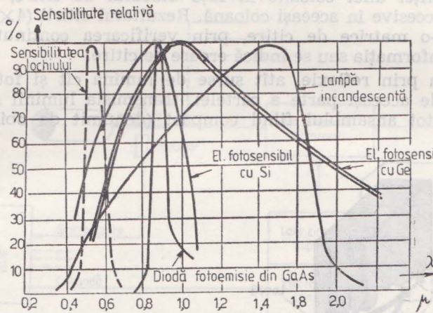
Fig. 5.4. Sensibilitatea elementelor fotoelectrice.
