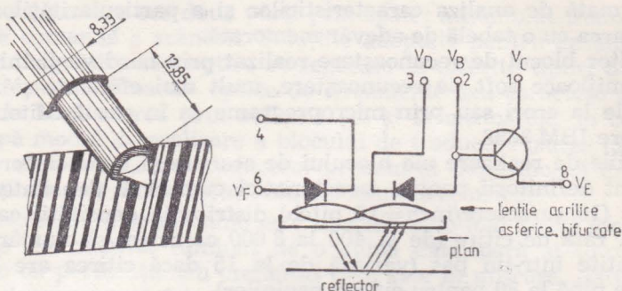
Fig. 9.3. Sesizor reflectiv de mare rezoluție HEDS-1000 (Hewlett-Packard):
