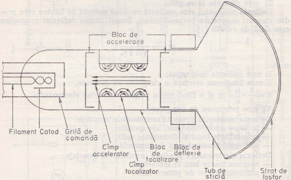
Fig. 7.1. Schema tubului cu vid cu explorare periodică (CRT).
