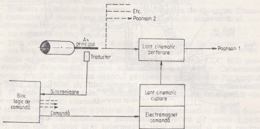
Fig. 5.7. Schema mecanismului de perforare.
