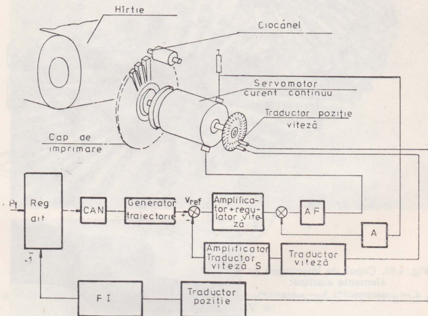
Fig. 4.66. Schema sistemului de selectare a caracterului prin servopозиționarea capului de imprimare.
